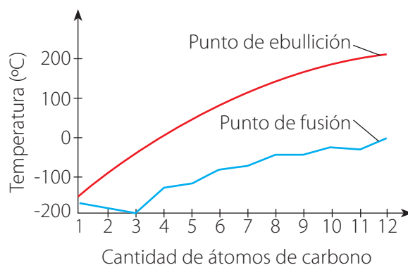
Gráfico n° 1. Puntos de fusión y ebullición de alcanos alifáticos
