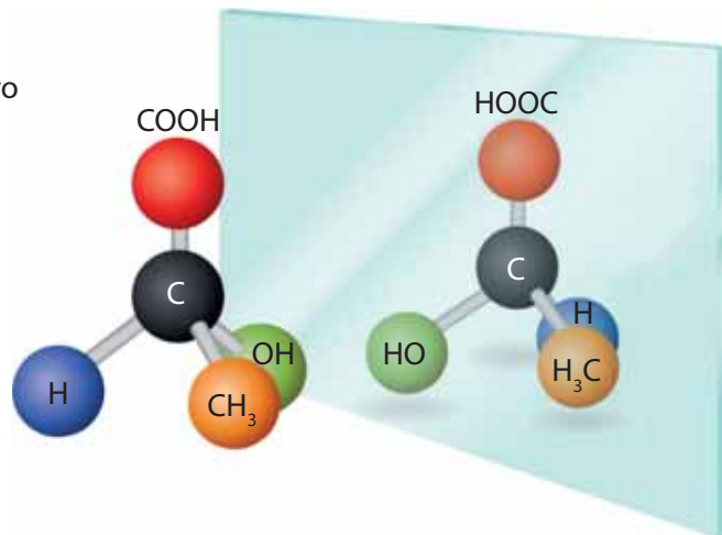
Enantiómeros del ácido láctico.
