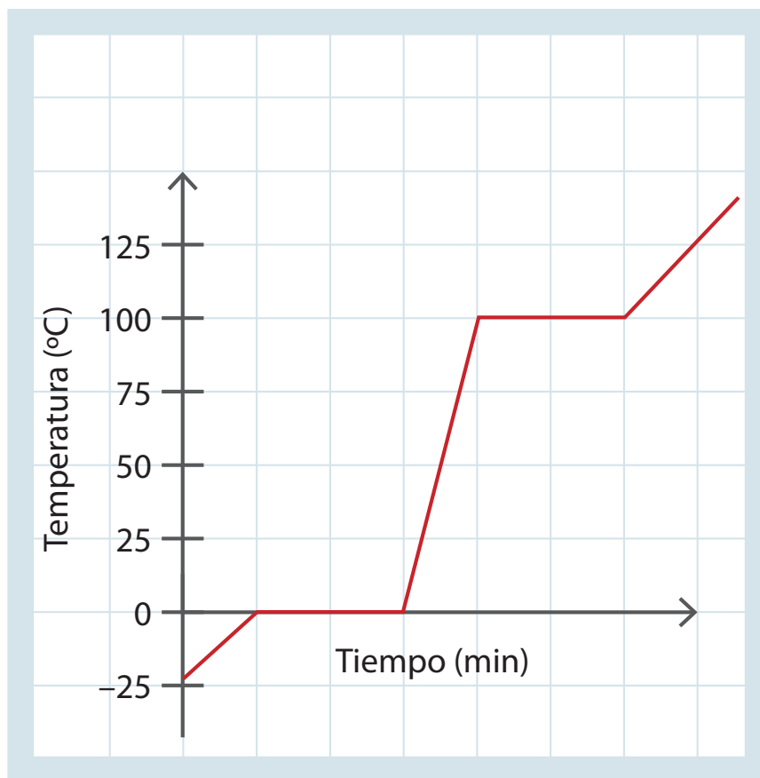
Gráfico n° 9: Comportamiento térmico del agua
